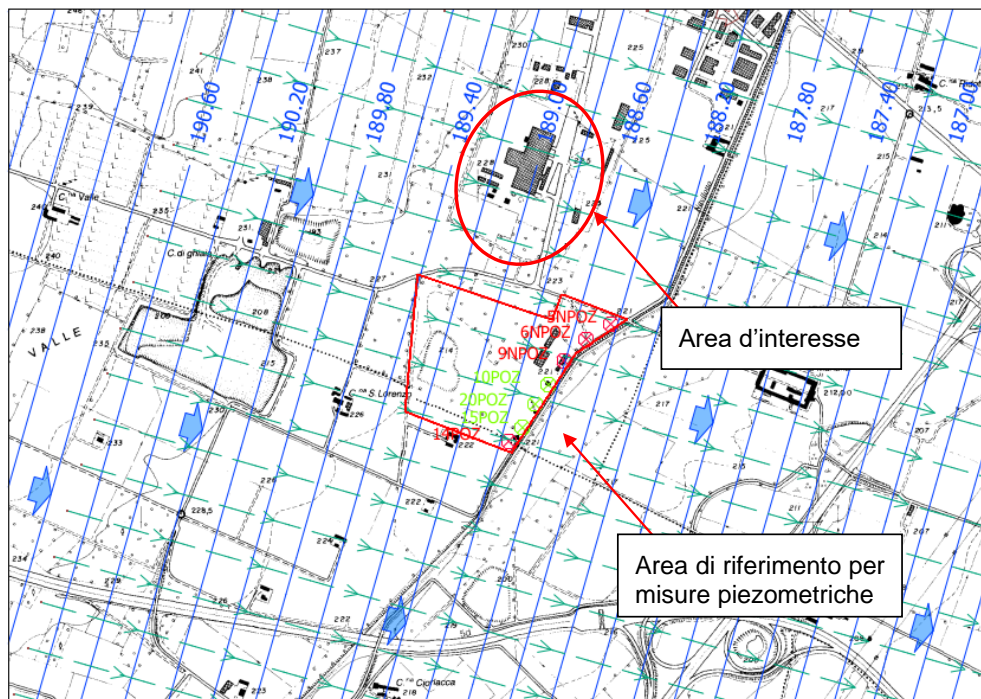
Figura 5.2b Piezometria statica alla minima escursione (Fonte: Relazione geologica)
