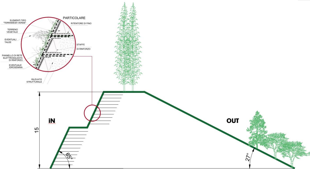
Figura 3234 - Sezione tipologica della collina realizzata con terre armate e terre da riporto
