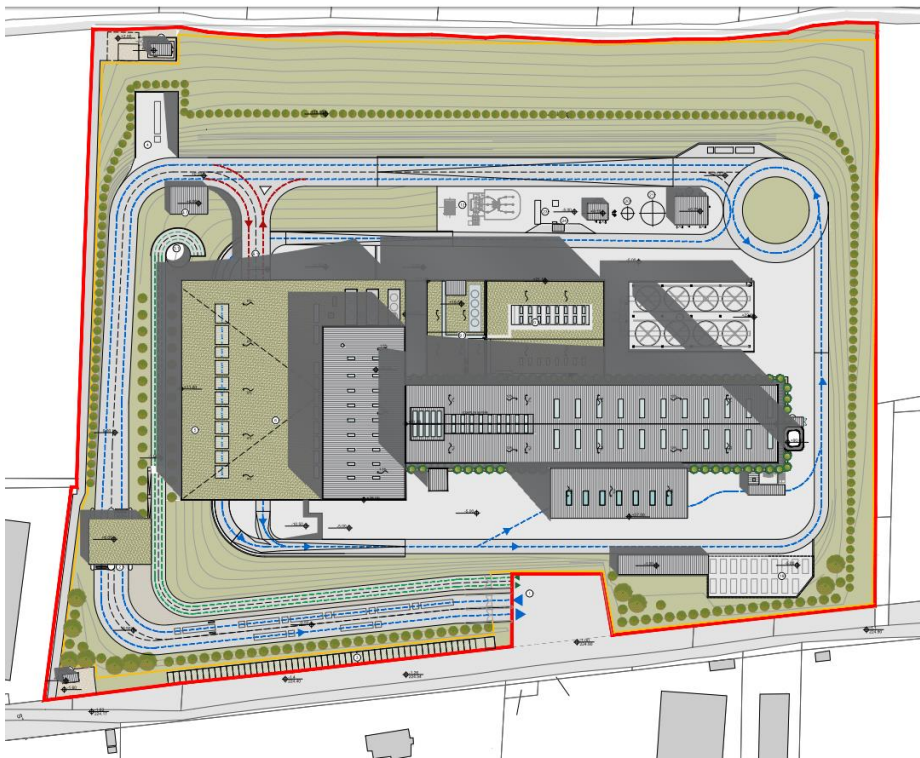
Figura 3130 - Pianta della copertura dell'impianto con coperture verdi
