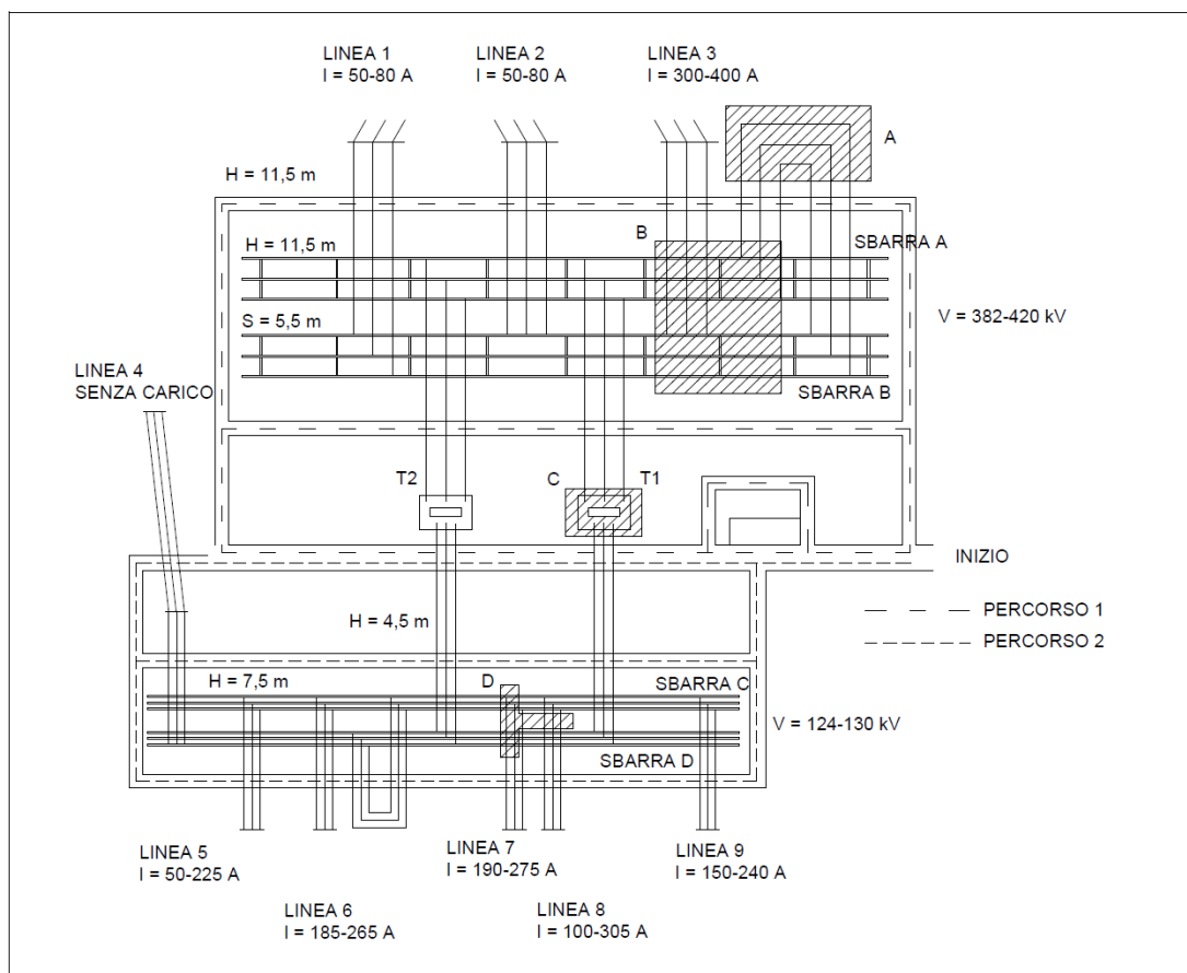
Fig. 1 – Pianta di una tipica stazione 380/132 kV con l'indicazione delle principali distanze fase-fase (S) e fase-terra (H) e delle variazioni delle tensioni e delle correnti durante la fase di misurazioni di campo elettrico e magnetico.
