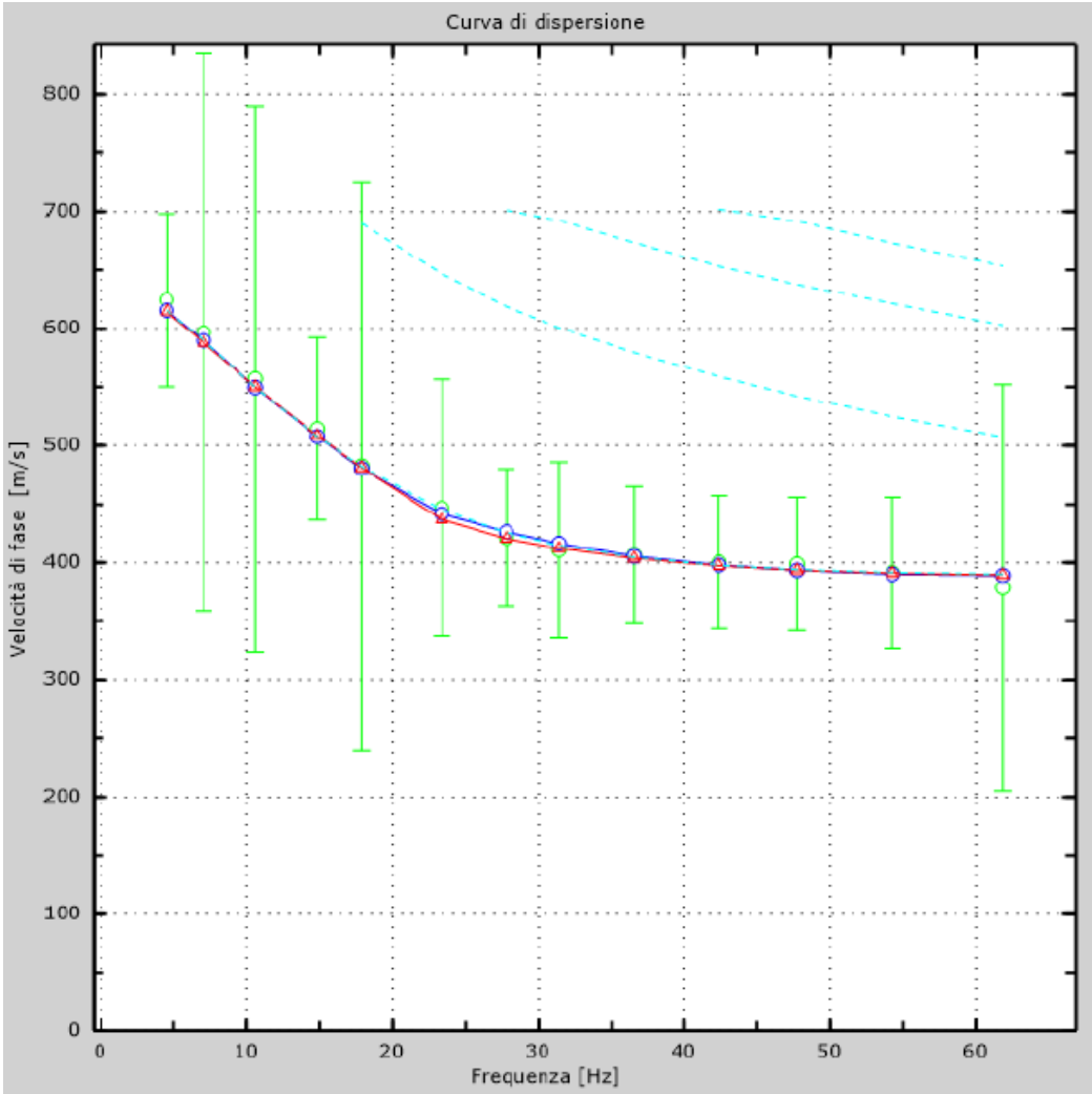
Figura 49: Velocità numeriche (Punti sperimentali - verde, modi di Rayleigh - ciano, curva apparente - blu, curva numerica – rosso)
