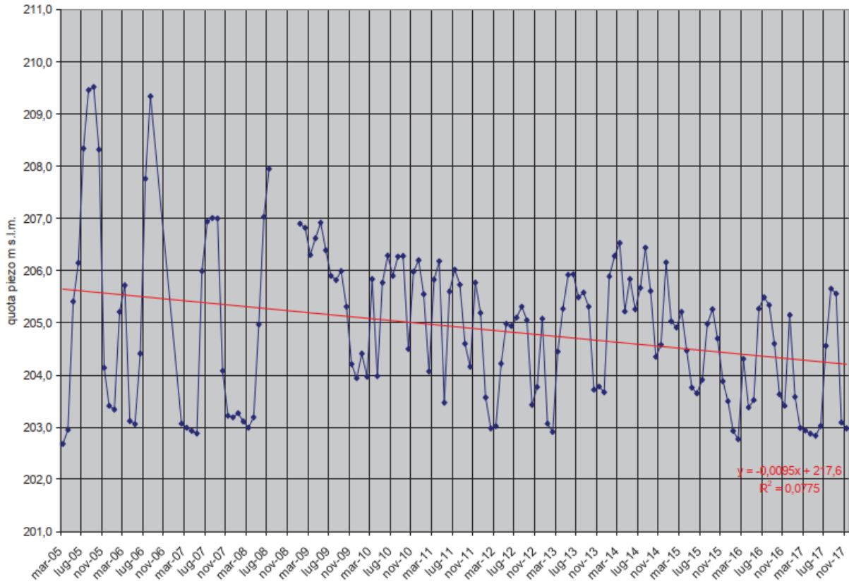
Figura 30: Trend piezometrico piezometro PII13
