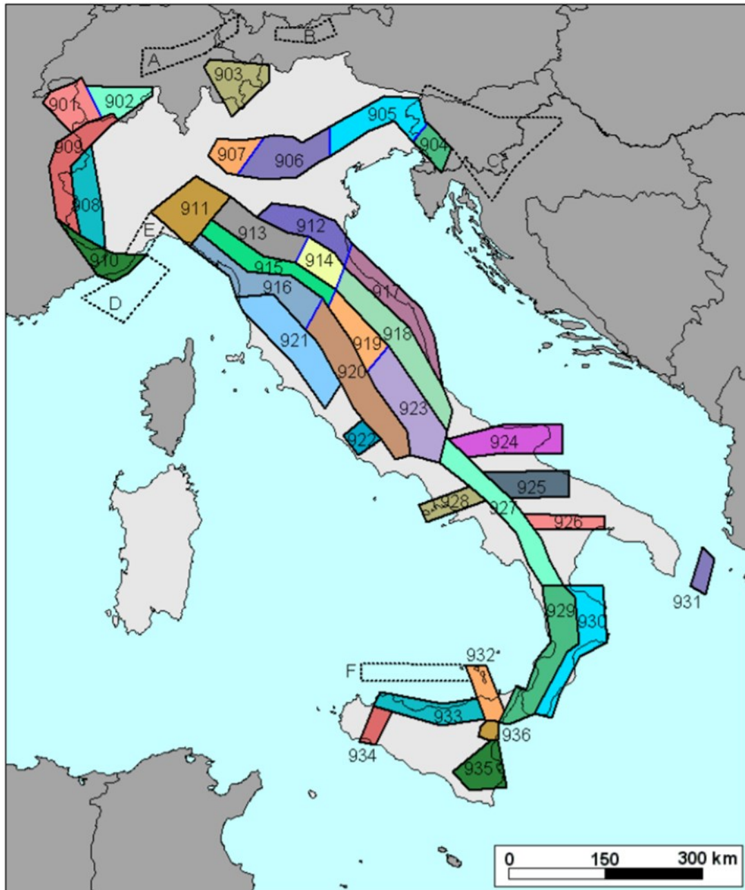
Figura40: sismogenetica ZS9
