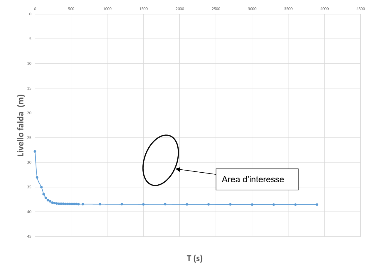
Figura 18: - 07/10/91 - Pozzo 4 - Prova 1 (Emungimento)
