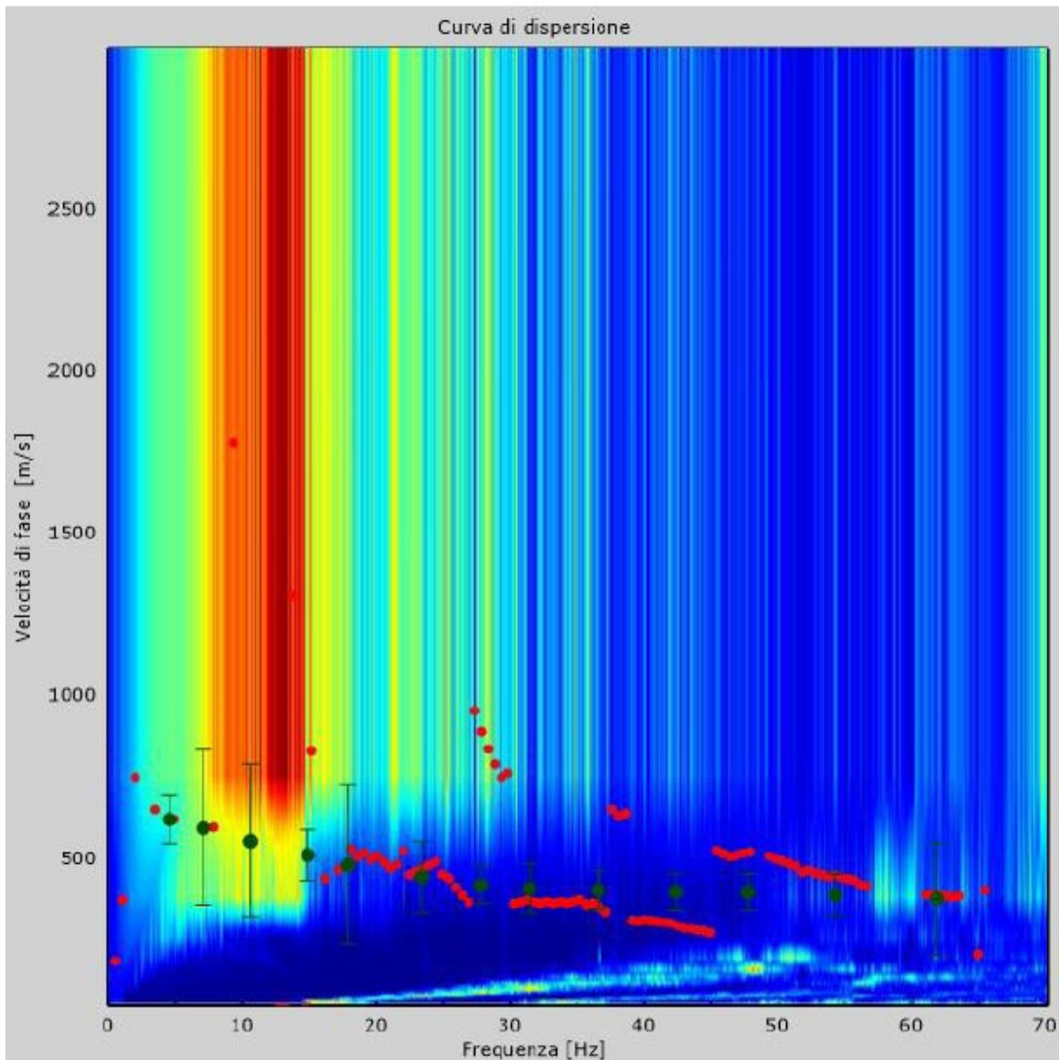
Figura 50: Curva di dispersione sperimentale
