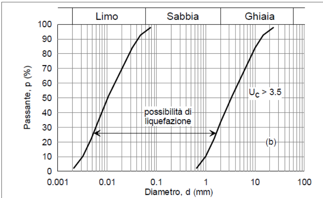
Figura 60: Figura 7.11.1 NTC 2018-Fuso granulometrico di terreni suscettibili di liquefazione.
