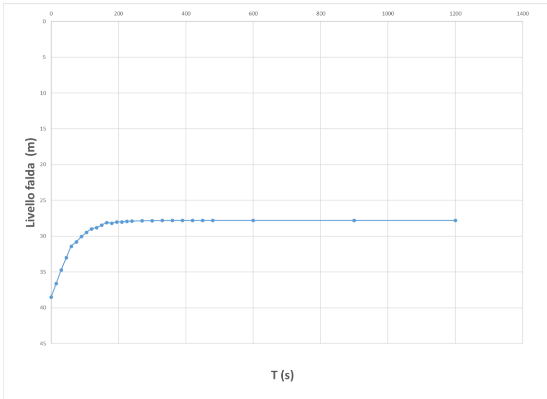
Figura 19: - 07/10/91 - Pozzo 4 - Prova 2 (Risalita)
