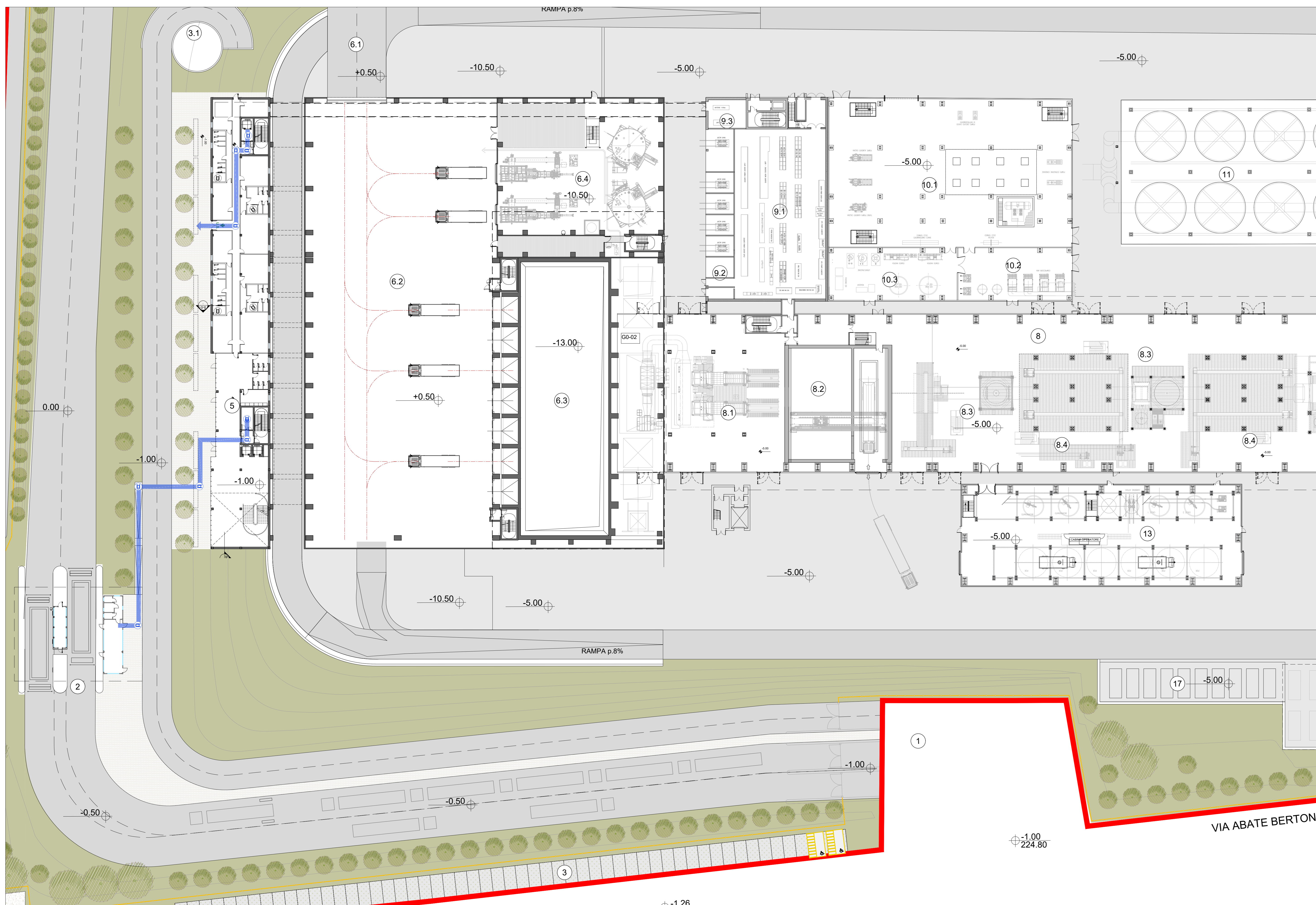
Planimetria Generale piano terra Scala 1:350
