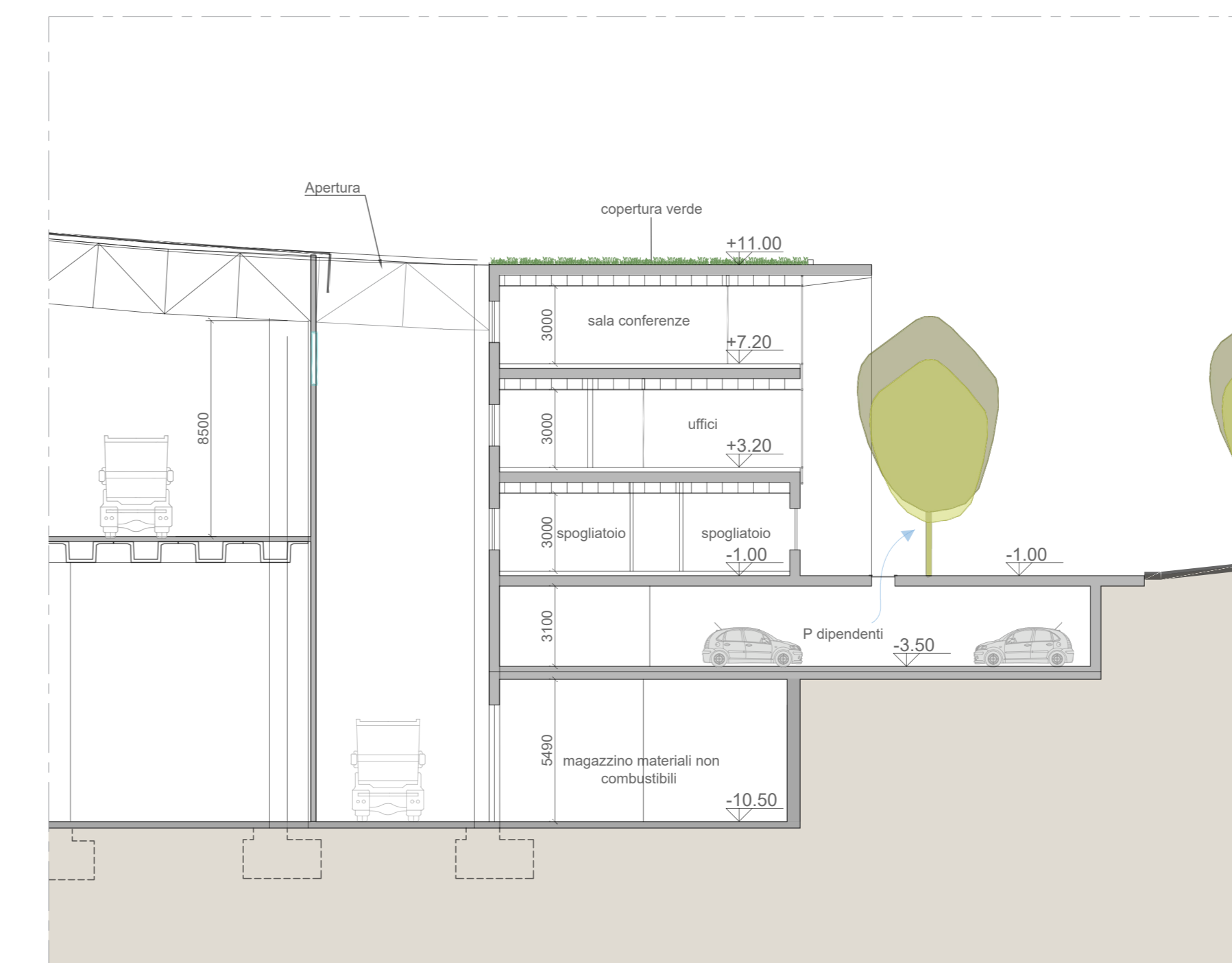
Sezione trasversale S1 Scala 1:200
