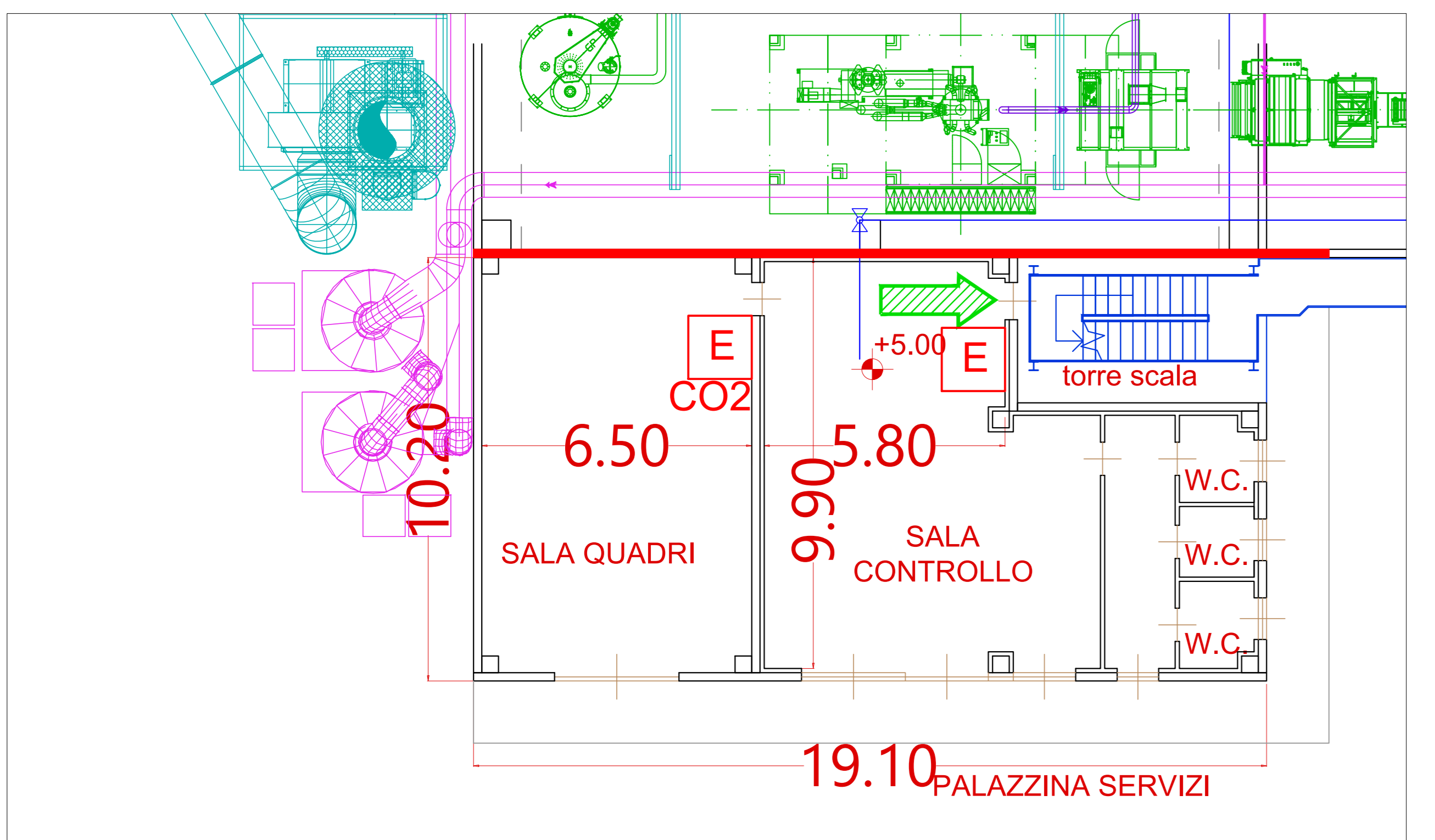
PIANTA PALAZZINA SERVIZI PIANO PRIMO
