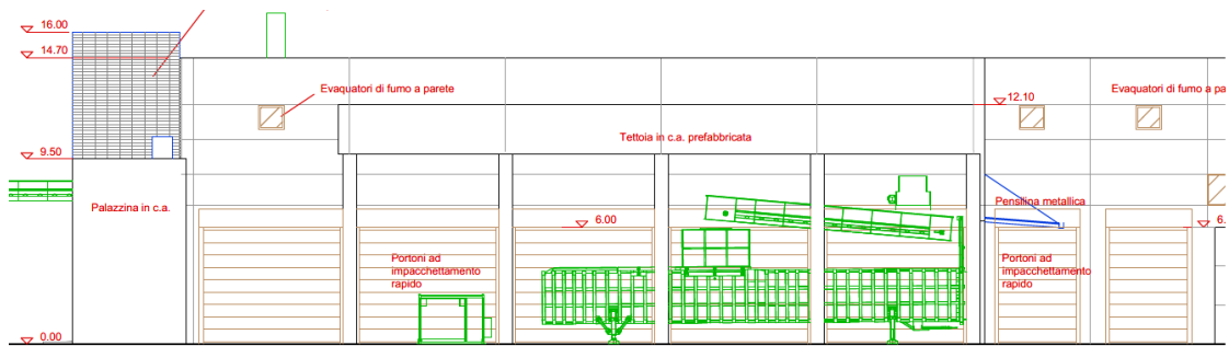
PROSPETTO OVEST
