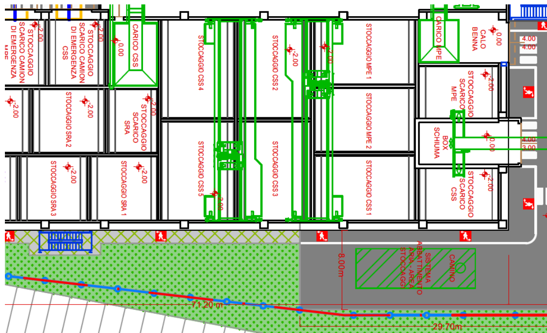
Figura 28: Sistema di abbattimento aria presentato con Permesso di costruire – Impianto SRA - Pianta
