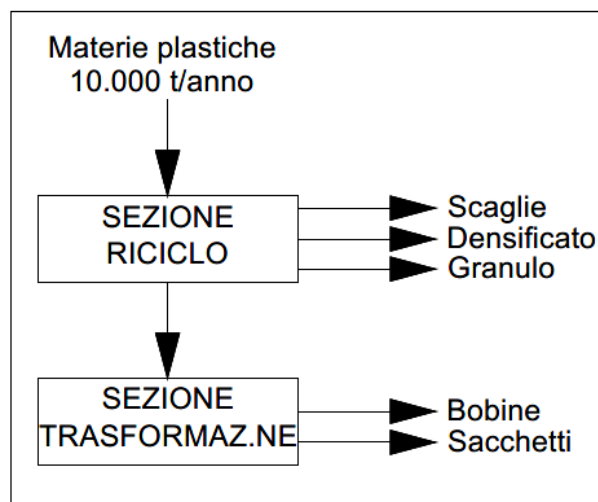
Figura 12: Schema semplificato Impianto di riciclo e produzione sacchetti
