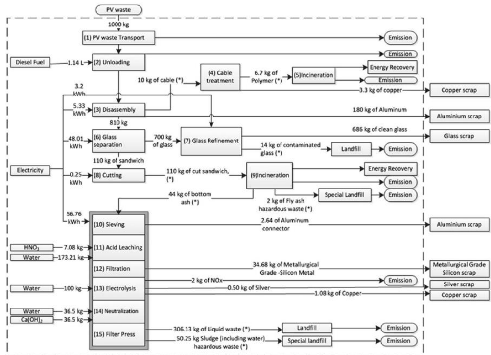
Figura 9 - Diagramma di flusso relativo al trattamento dei rifiuti da fotovoltaico (Fonte: Latussa C.L. et al.2016a) 31
