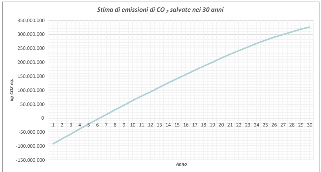
Figura 10 – Stima di risparmi di CO 2 nei 30 anni di vita dell'impianto fotovoltaico
