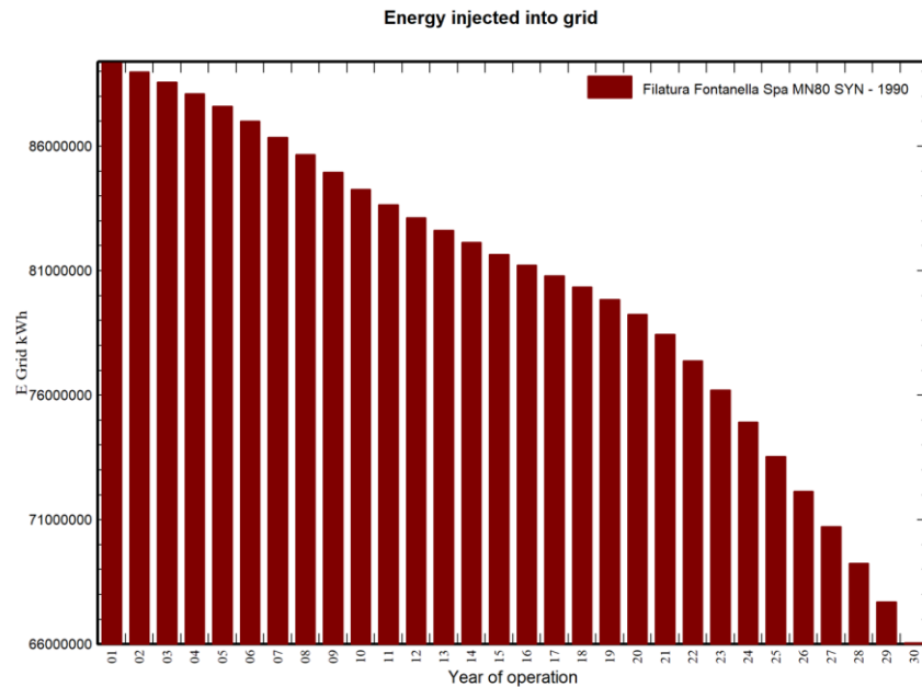
Figura 5 - Energia immessa in rete nei 30 anni di vita dell'impianto -Dati esportati dal software di calcolo PVSyst
