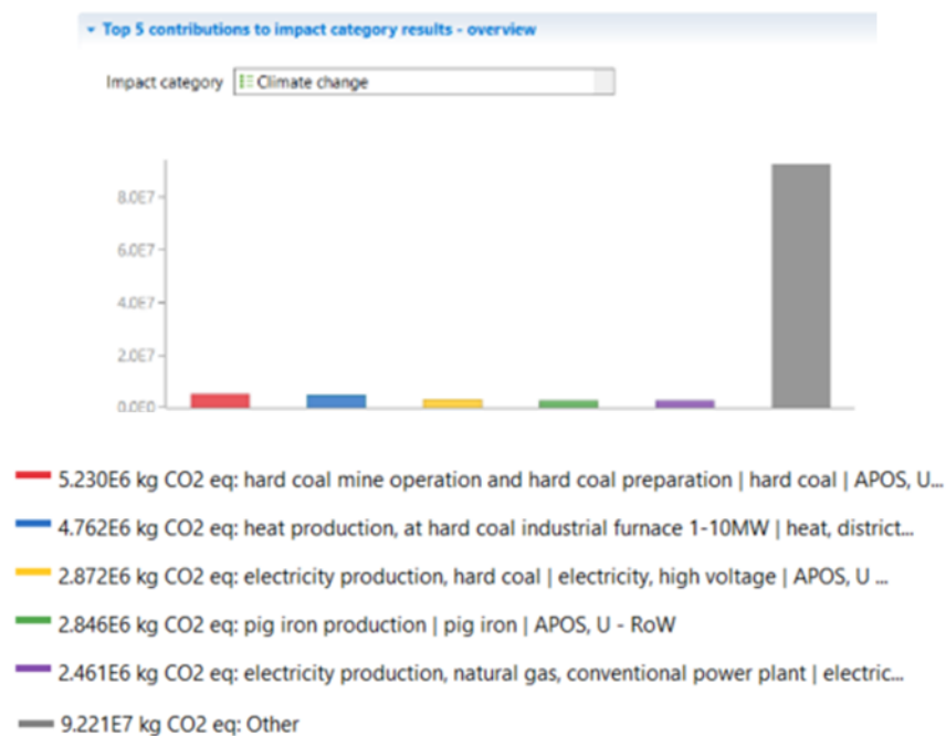
Figura 6 - Top 5 processi che incidono di più all'interno della categoria di impatto Climate Change
