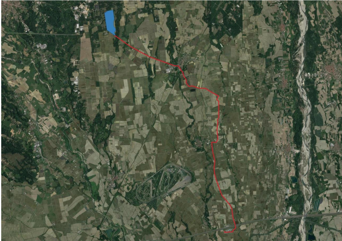
Localizzazione dell'opera; in blu, l'area destinata a campo fotovoltaico, in rosso il tracciato della linea a cavidotto/linea aerea
