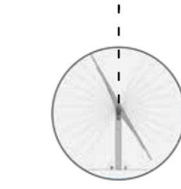
L'asse di vista dal Santuario verso i tracker dell'impianto è perpendicolare alla rotazione dei pannelli. Il riflesso dei vetri non risulta visibile a nessuna ora e variazione di rotazione della strutture.
