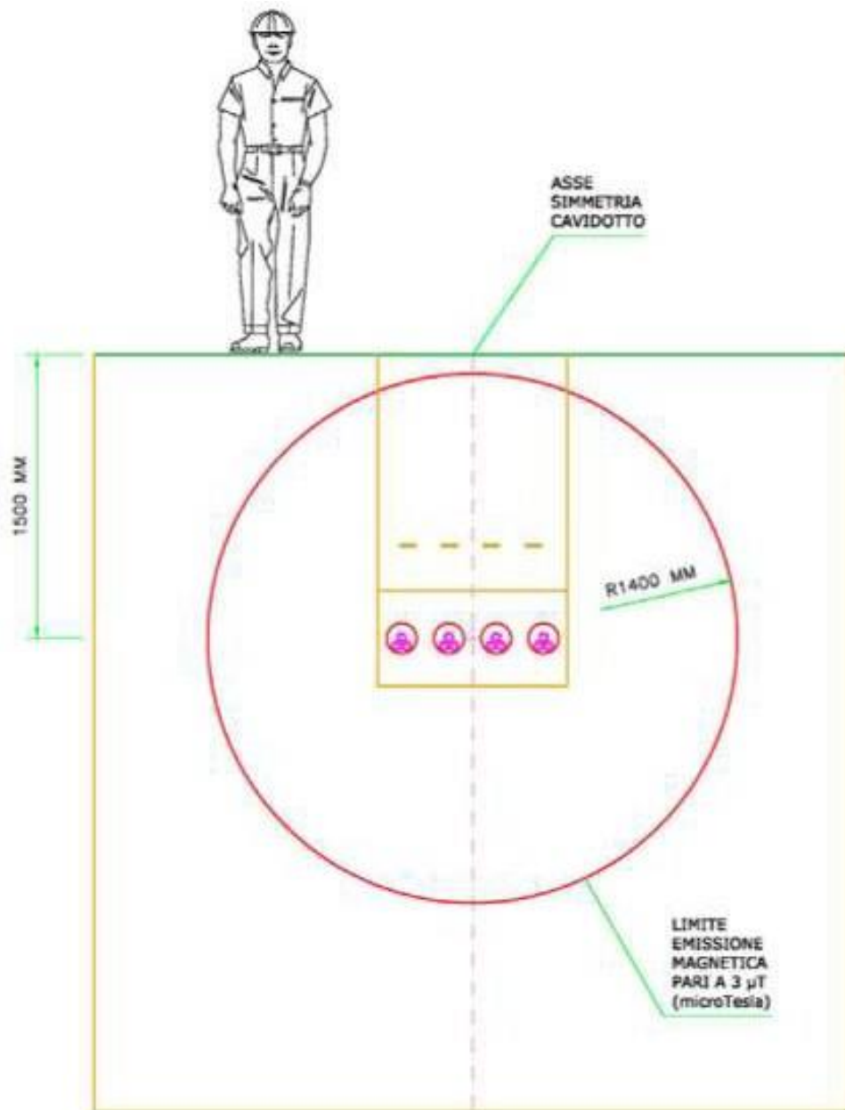
Figura 40 Volume di rispetto per il campo magnetico di una linea MT in cavo elicordato interrata.
