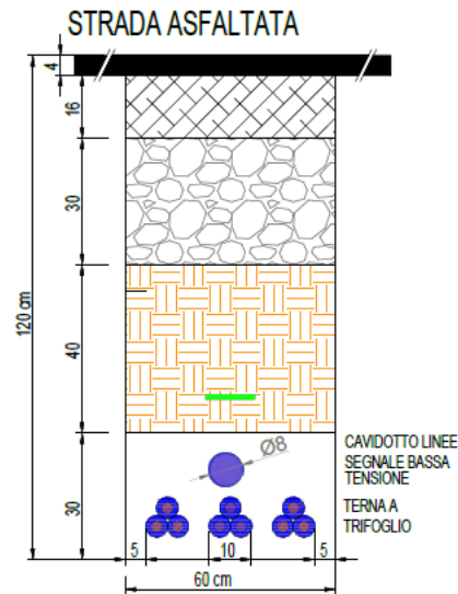
Figura 41 Sezione tipica di posa della linea in cavo su sede stradale per triplo cavidotto in MT
