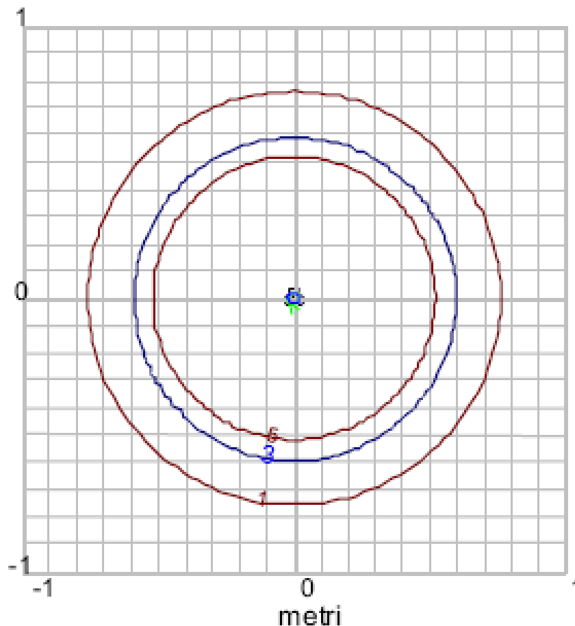
Figura 39 Curve di equilivello per il campo magnetico di una linea MT in cavo elicordato interrata (dalla Norma CEI 106-11)
