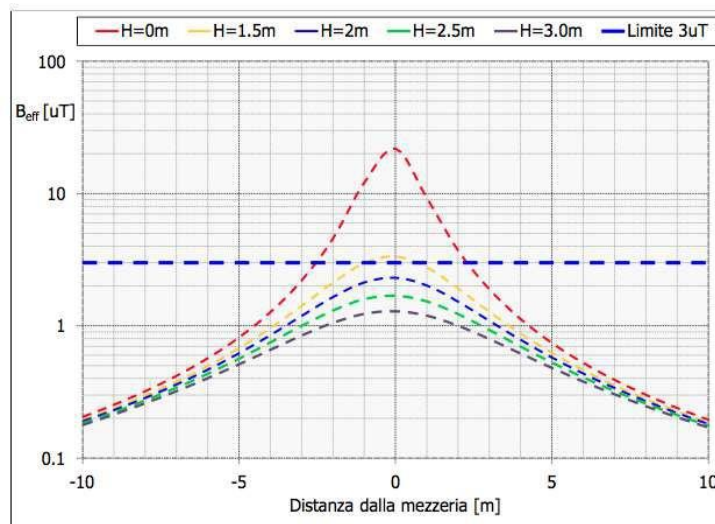
Figura 42 Andamento dell'induzione magnetica prodotta dalla linea in cavo per la massima corrente del cavo
