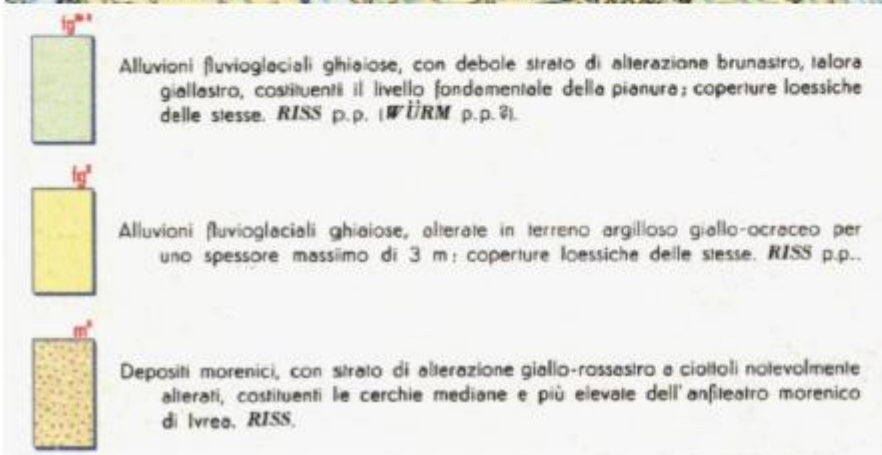
Figura 30 Carta geologica
