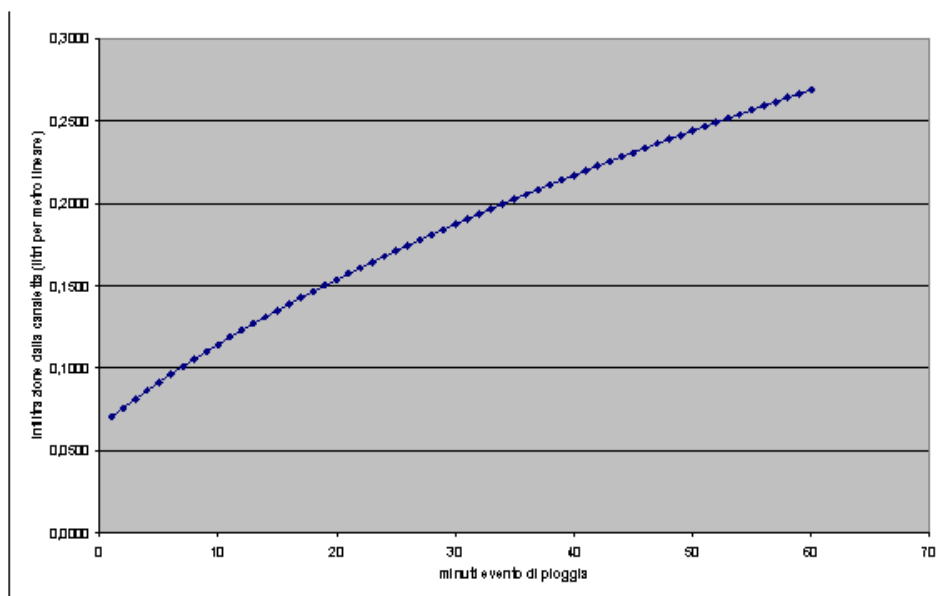
Andamento della portata di infiltrazione durante la pioggia di progetto
