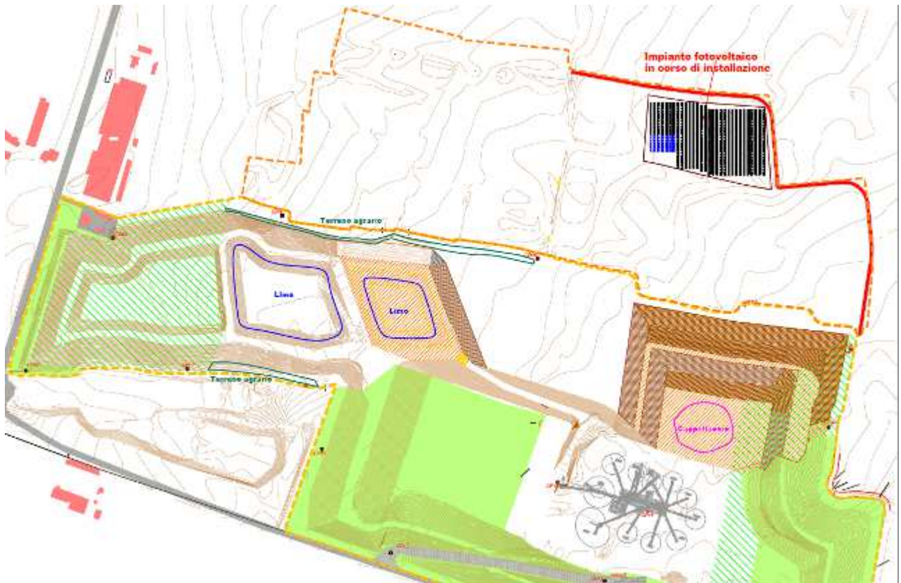
Installazione iniziale - ubicazione dell'impianto
