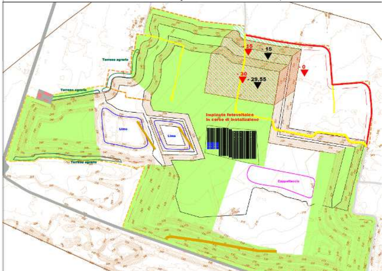
Spostamento dell'impianto fotovoltaico in corrispondenza della fase 4 di scavo all'interno dell'area di ampliamento
