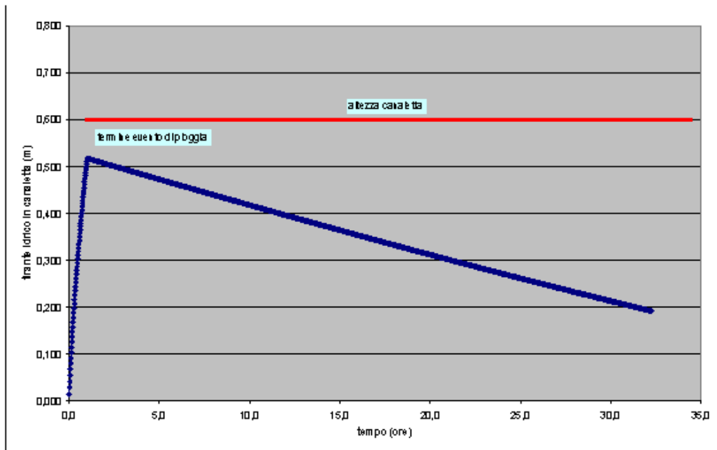
Andamento del tirante idrico all'interno della canaletta di fondo
