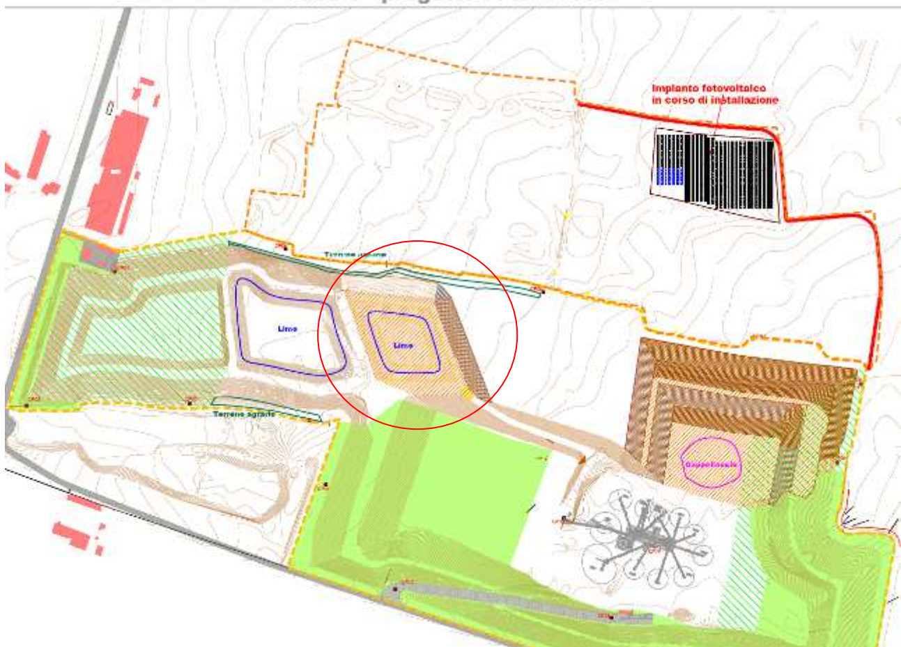
Fase 3 - progetto autorizzato
