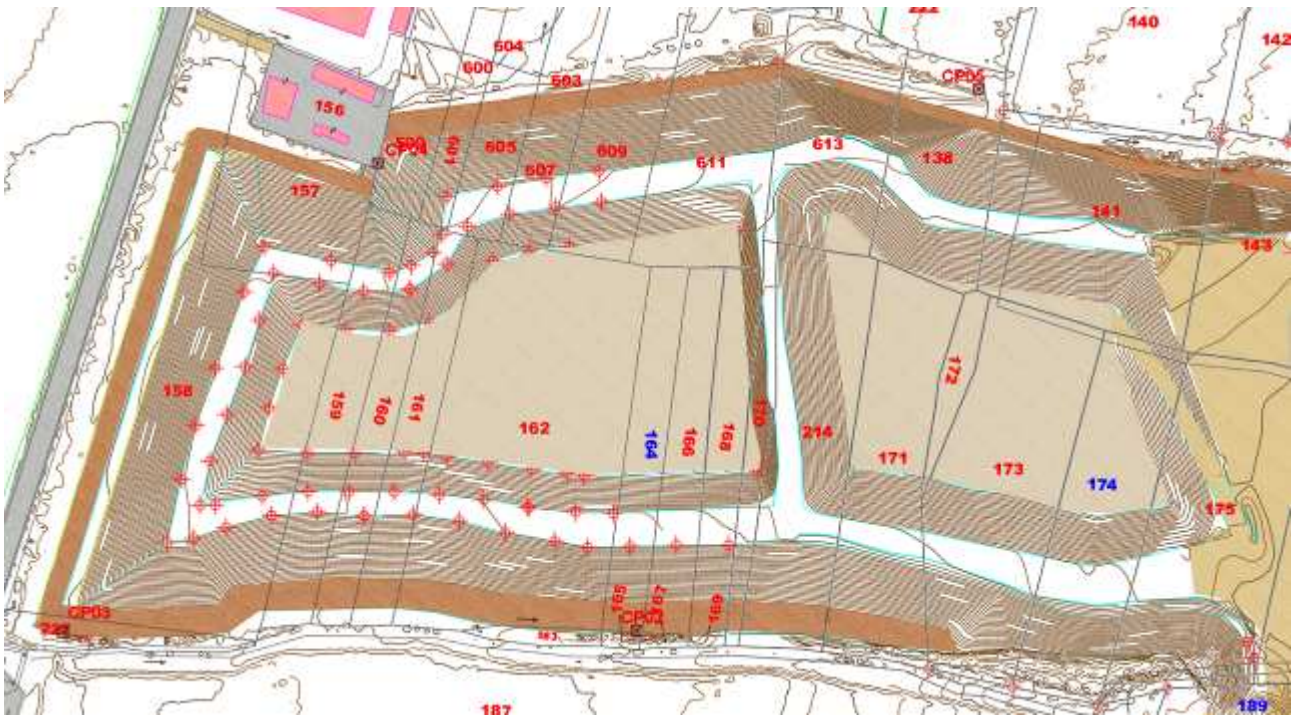
Tav. 05 Planimetria stato attuale – vasche di sedimentazione – Area Ovest
