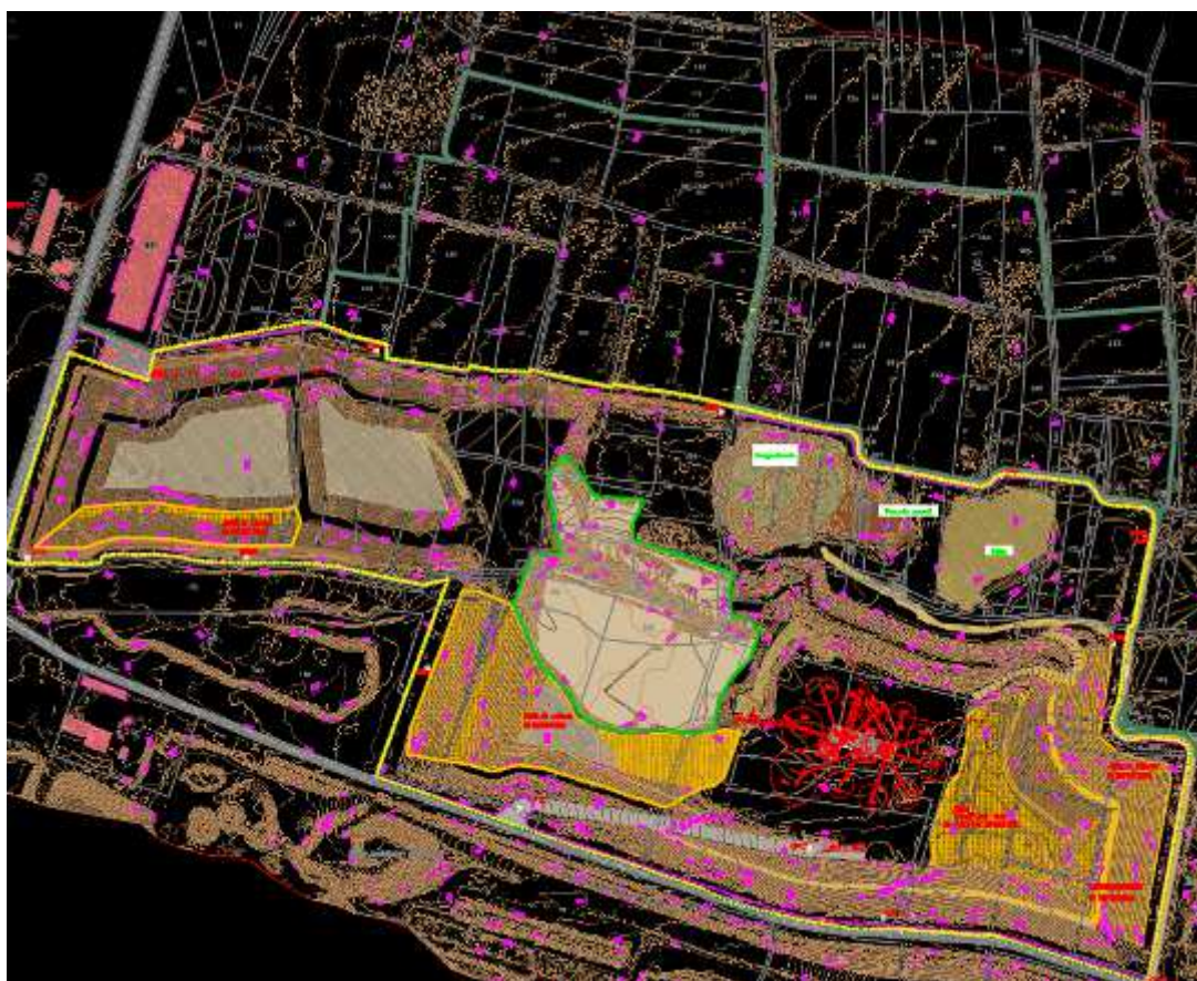
Tav. 05 Planimetria attuale
