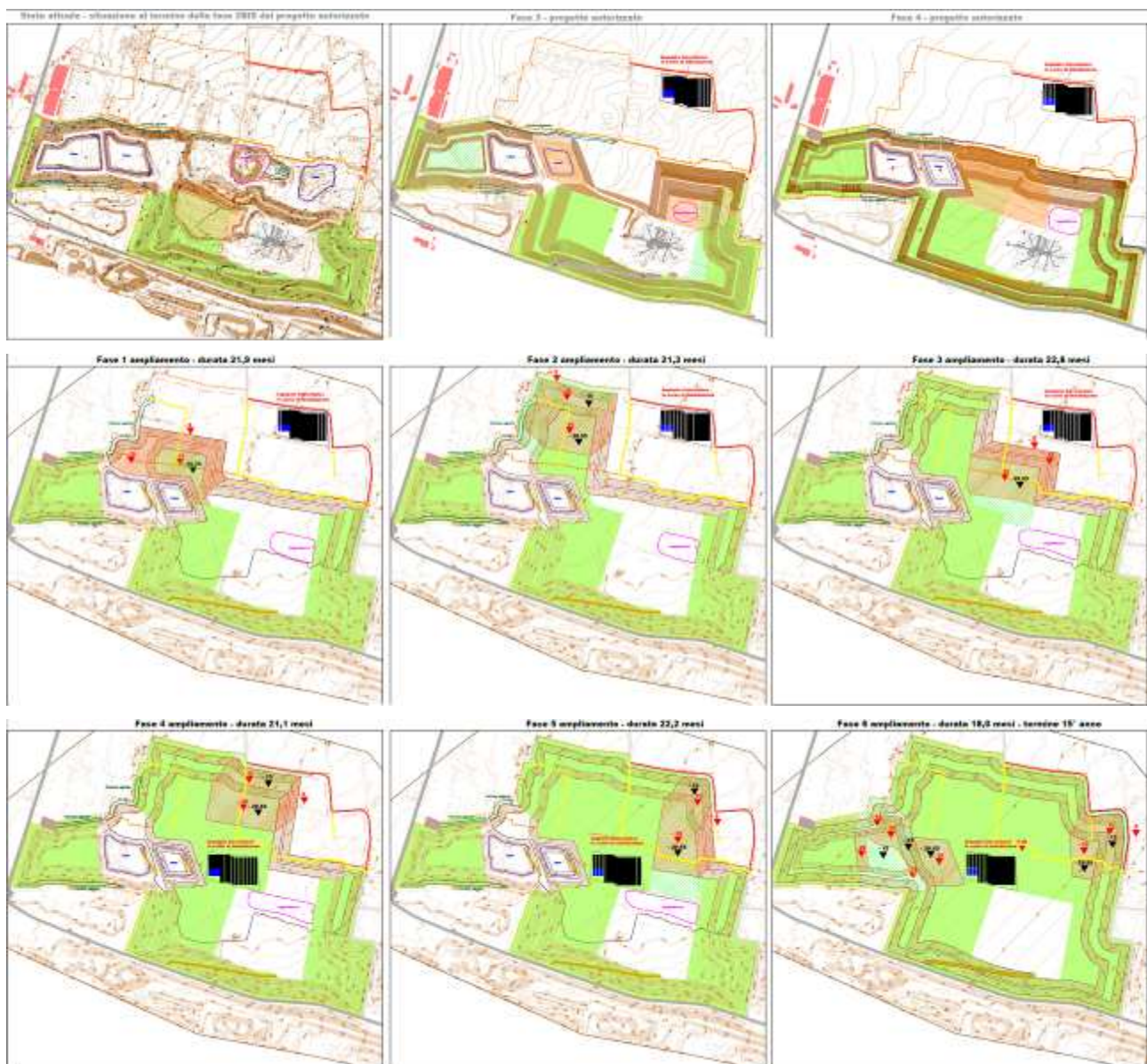
Tav. 07 Planimetria fasi
