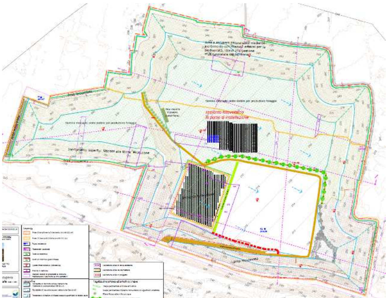
Tav. 10 planimetria finale ripristino
