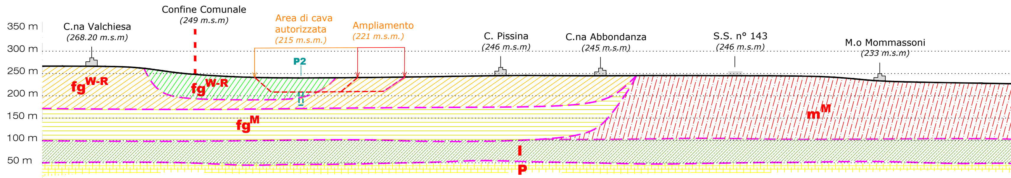
Sezione geologica strutturale NW-SE
