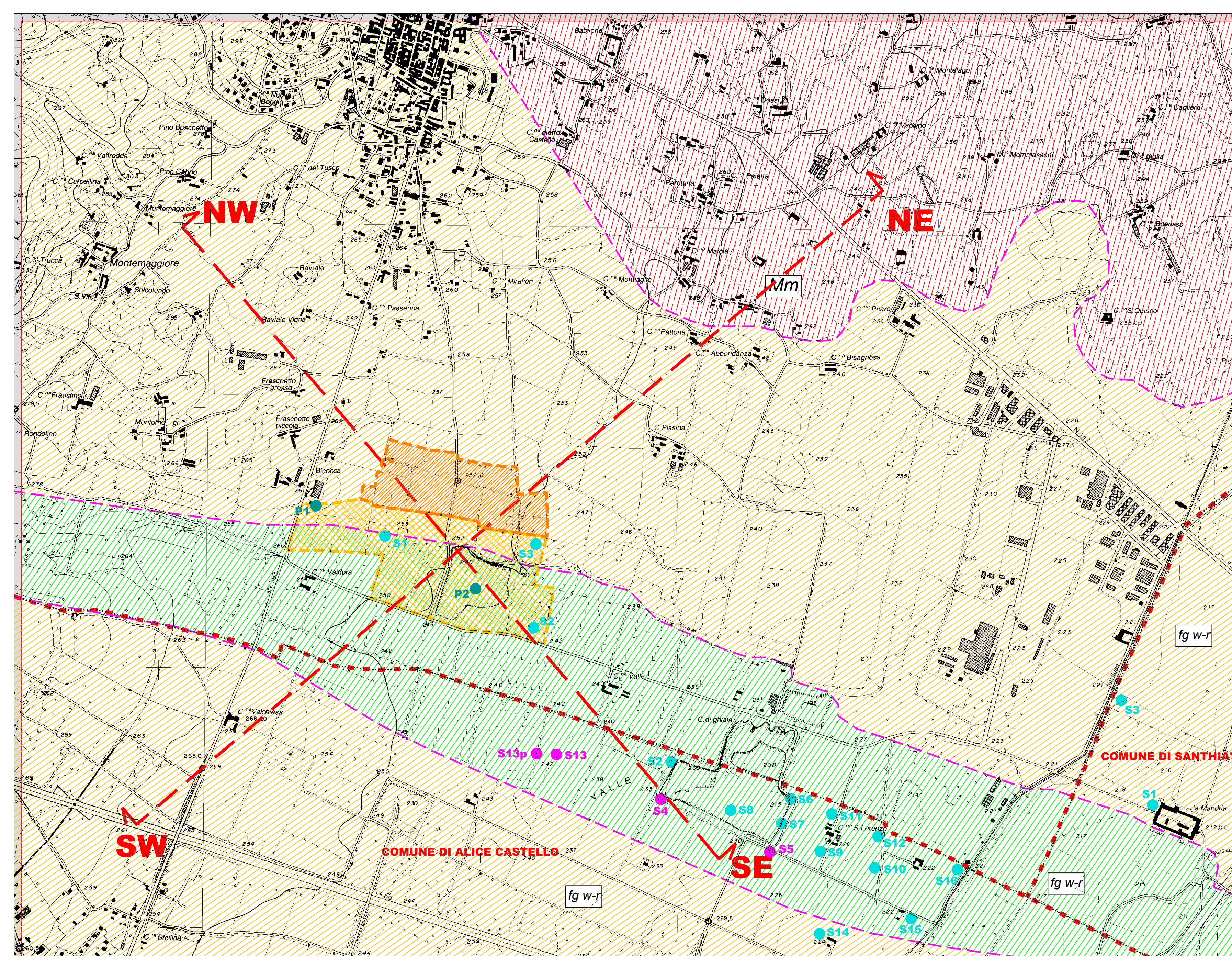
Sezione geologica strutturale SW-NE
