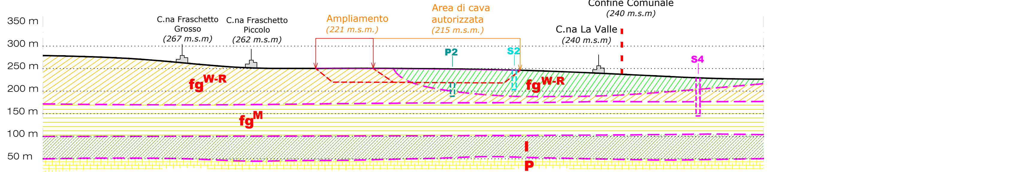
Sezione geologica strutturale NW-SE
