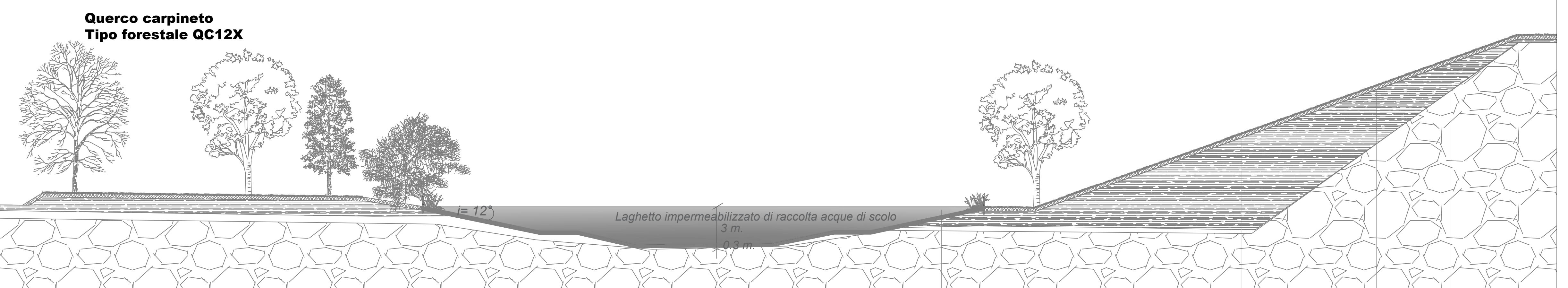
A - PARTICOLARE SEZIONE LAGHETTO - Scala 1:200.-
