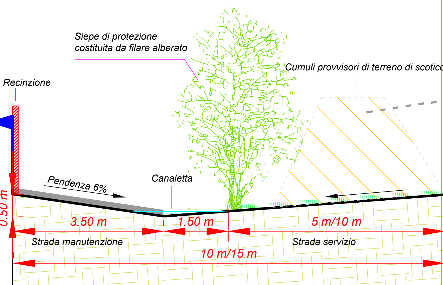
PARTICOLARE DEL FASCIA DI RISPETTO - Scala 1:50.-
