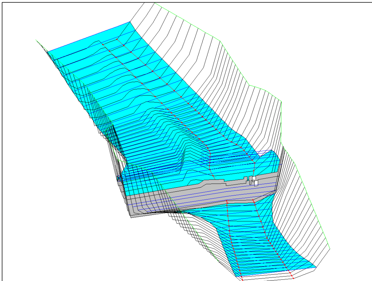
Figura 3.1 - La figura riporta la ricostruzione in tridimensionale dell'alveo del T. Concabbia nei pressi del sito di realizzazione dell'opera di presa.
