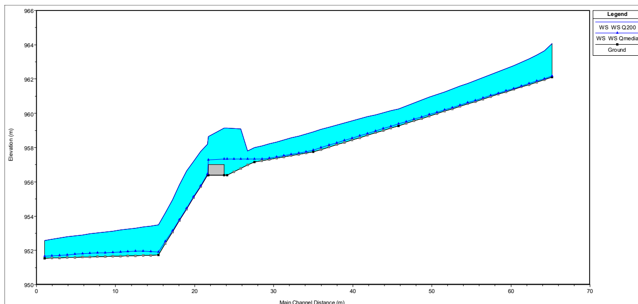
Figura 3.4- Profilo dell'alveo del Torrente Concabbia: Q200 e Qmedia.
