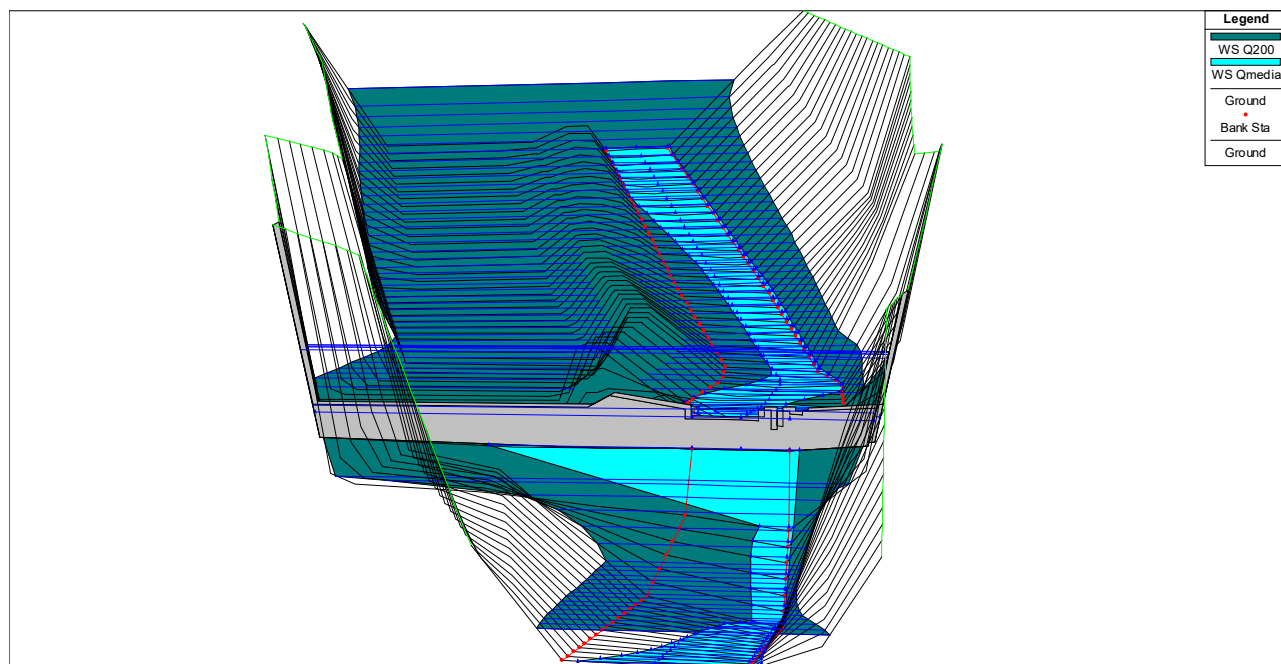
Figura 3.3– Area bagnata dell'alveo del Torrente Concabbia: Q200
