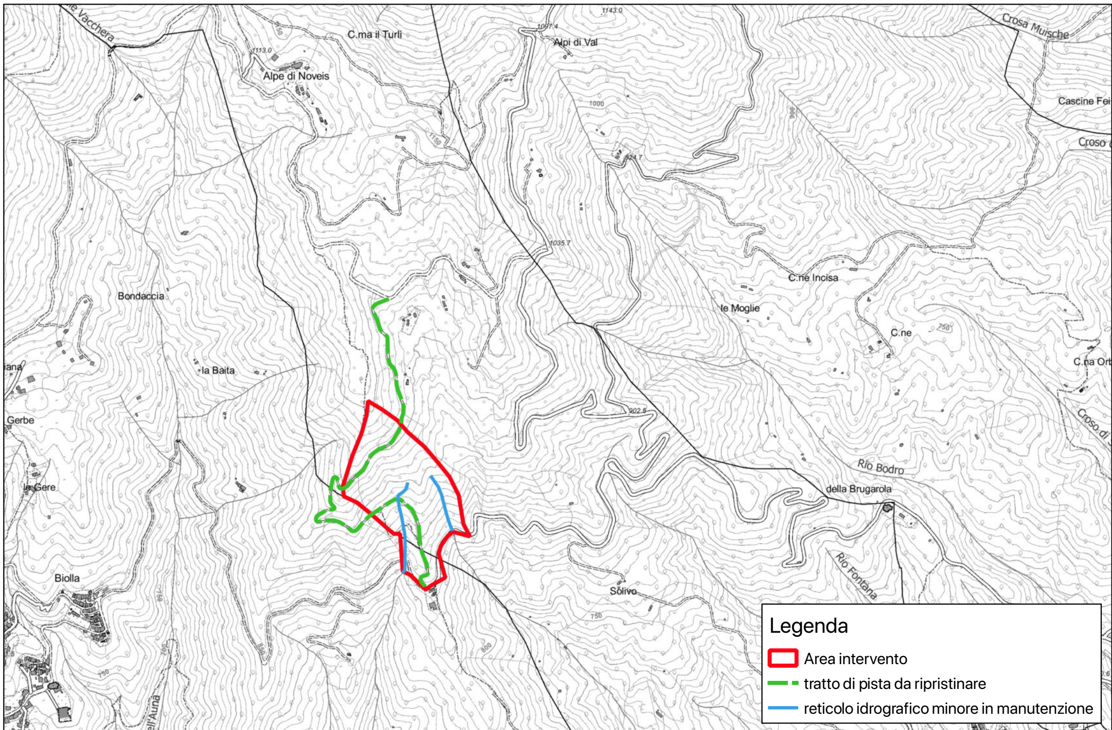
Bettoni 4.0/Edilcave - Trasformazione del bosco per attività estrattive Tavola 9 - Intervento Caprile Pian delle Rape Scala 1:10.000
