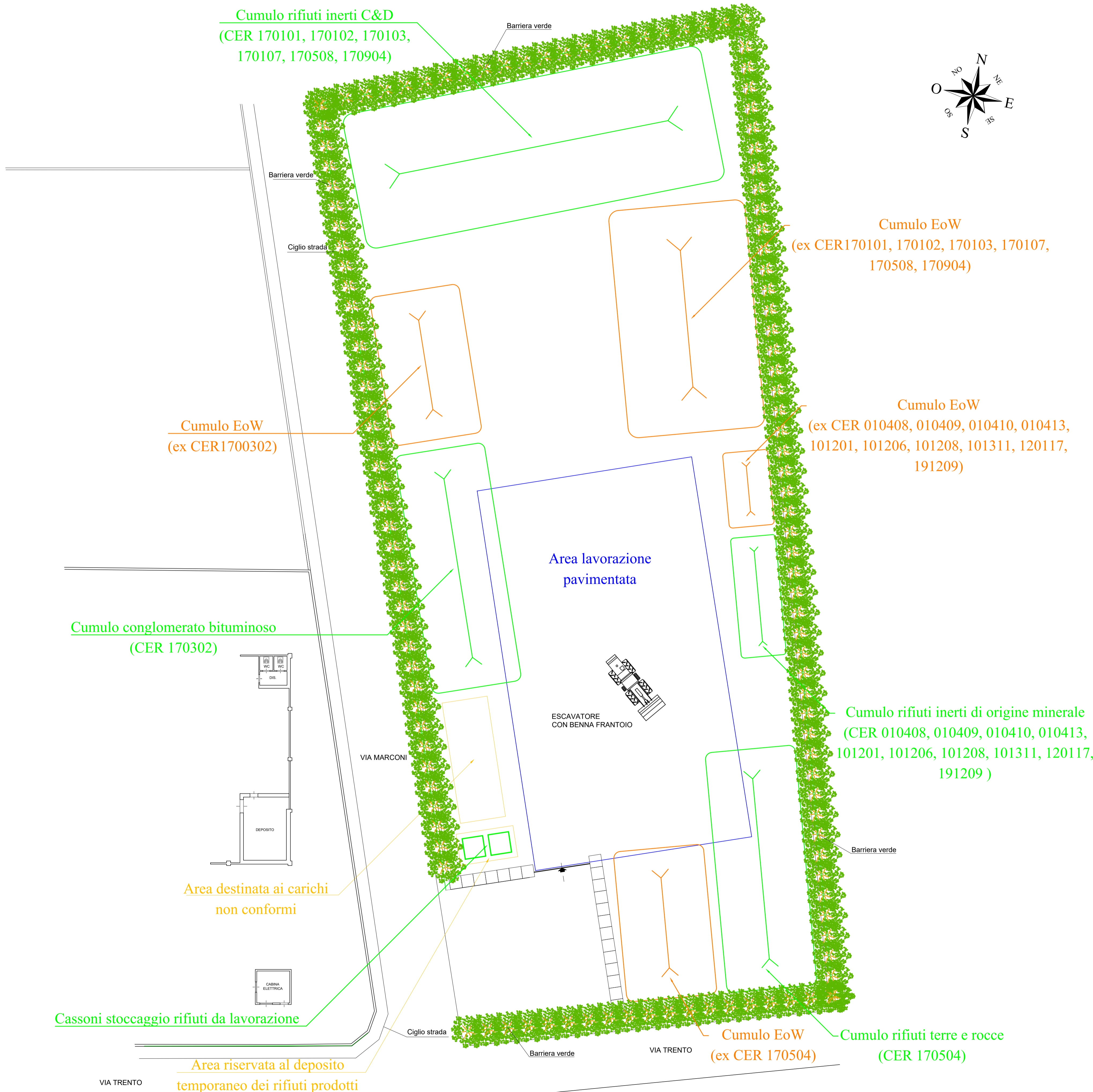
Layout impianto - Sede operativa Via Trento S.n.c. - Scala 1:200
